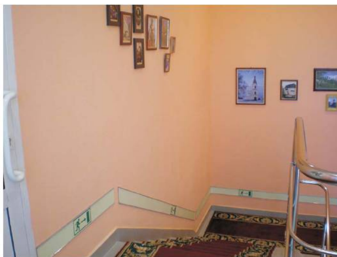
Рисунок А.5 - Вариант ФЭС с использованием направляющей линии шириной 100 мм и эвакуационных знаков направления движения
